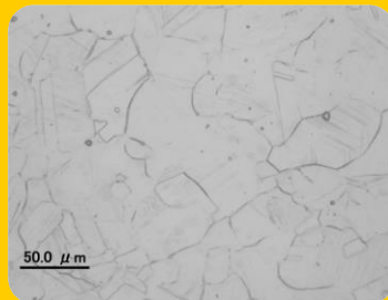
▲健全な金属組織
