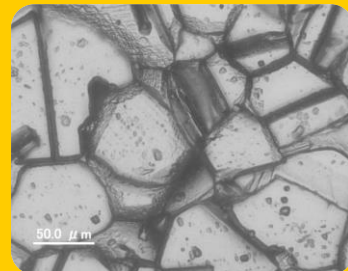
▲鋭敏化した金属組織
